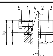
1 - прокладка; 2 - гайка; 3 - штуцер; 4 - кольцо уплотнительное; 5 – болт ВНИМАНИЕ! Болт 5 затягивать с усилием от 5 до 7 Н·м.
