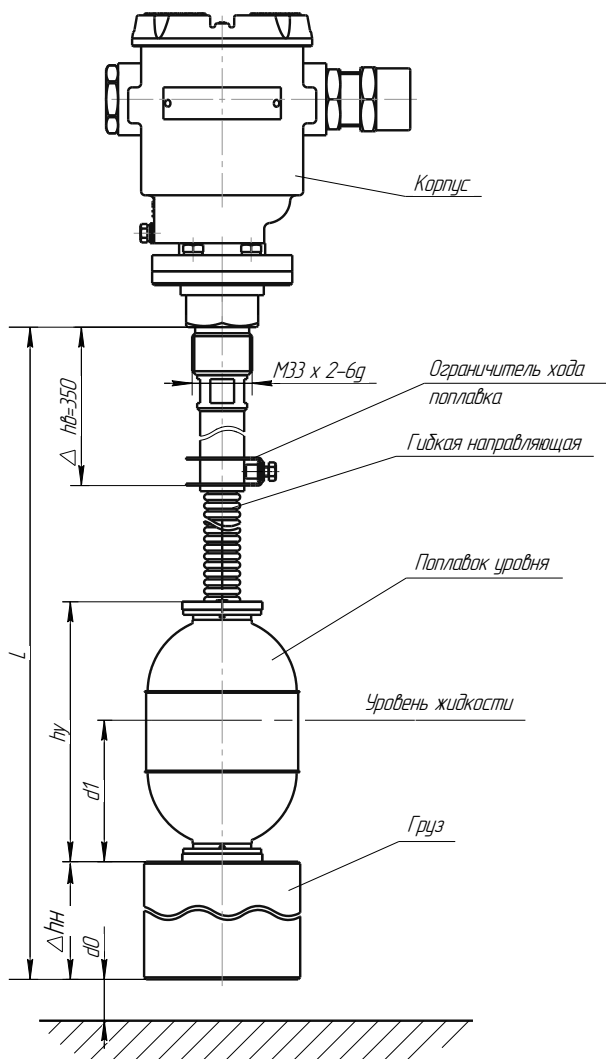
Рисунок 1 – Общий вид уровнемера
