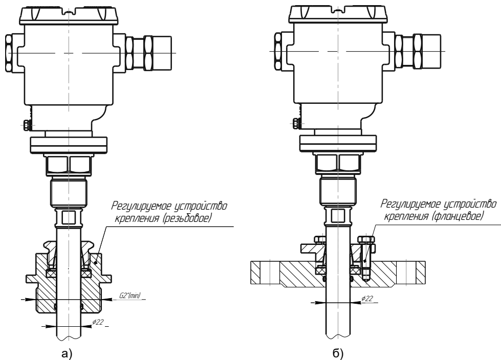
Рисунок 6. Регулируемое устройство крепления; а) резьбовое; б) фланцевое
