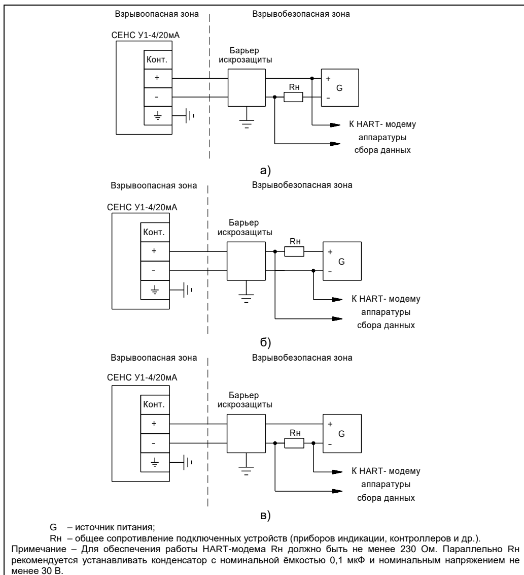
Рисунок 8 – Схемы подключения
