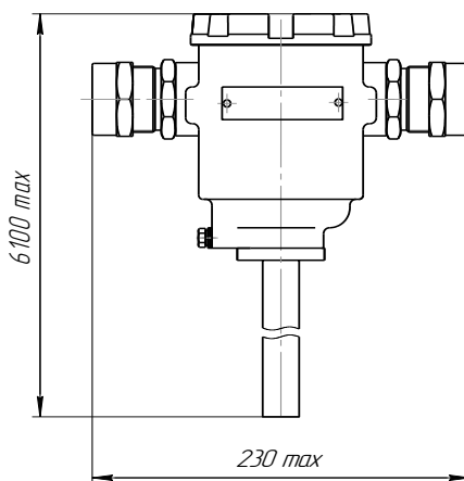
Рисунок 11 (лист 3 из 5) – Чертеж средств взрывозащиты
